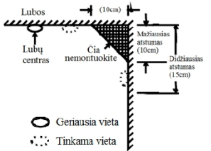
4 pav.: siūlomos vietos jutikliui montuoti
