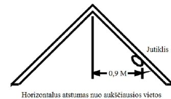
5 pav.: siūlomos vietos jutikliui montuoti, jeigu yra nelygios lubos
